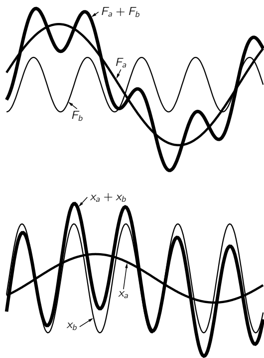
图 25.1: 线性系统叠加的一个例子
